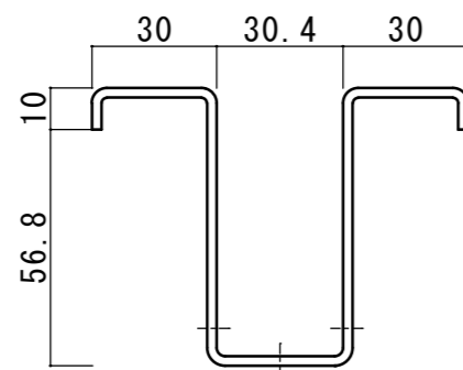
【正面図】
